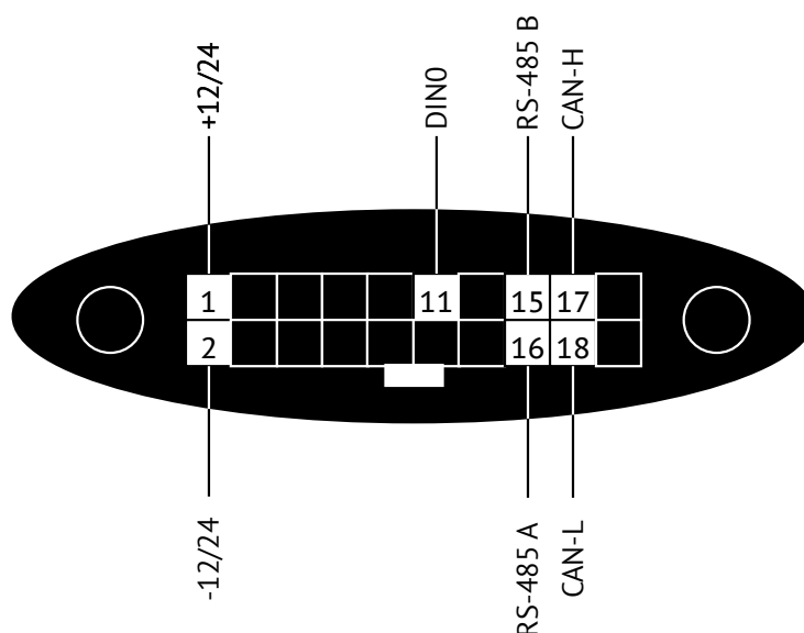
Рисунок 1 – 20-контактный разъём
