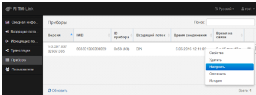
Рисунок 4. ПО RITM-Link
