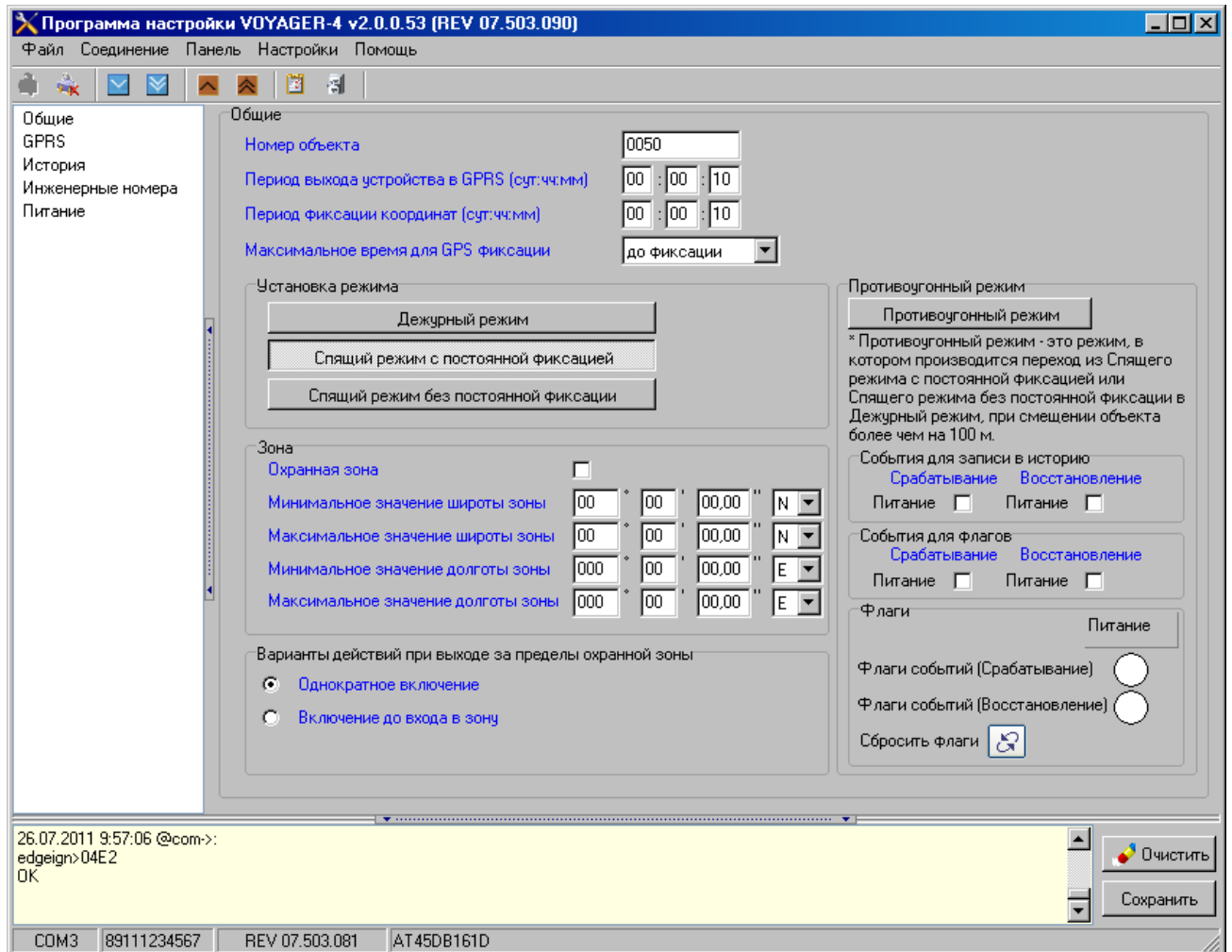
Рис.4.3.1.1. Страница общих настроек
