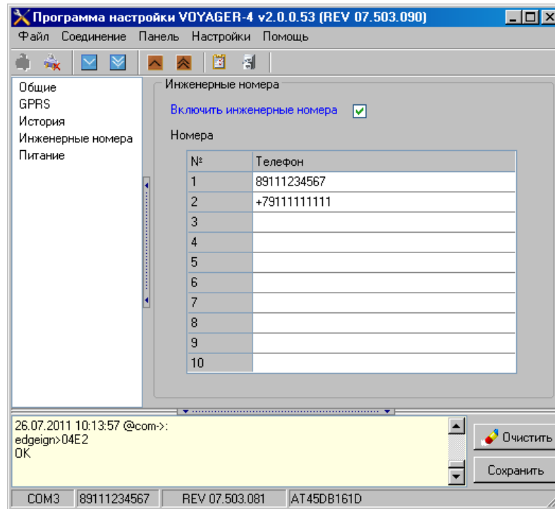
Рис. 4.3.5.1. Страница настройки инженерных номеров
