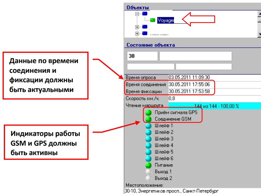
Рис. 5.1. Панель состояния объекта в программе PCN8
