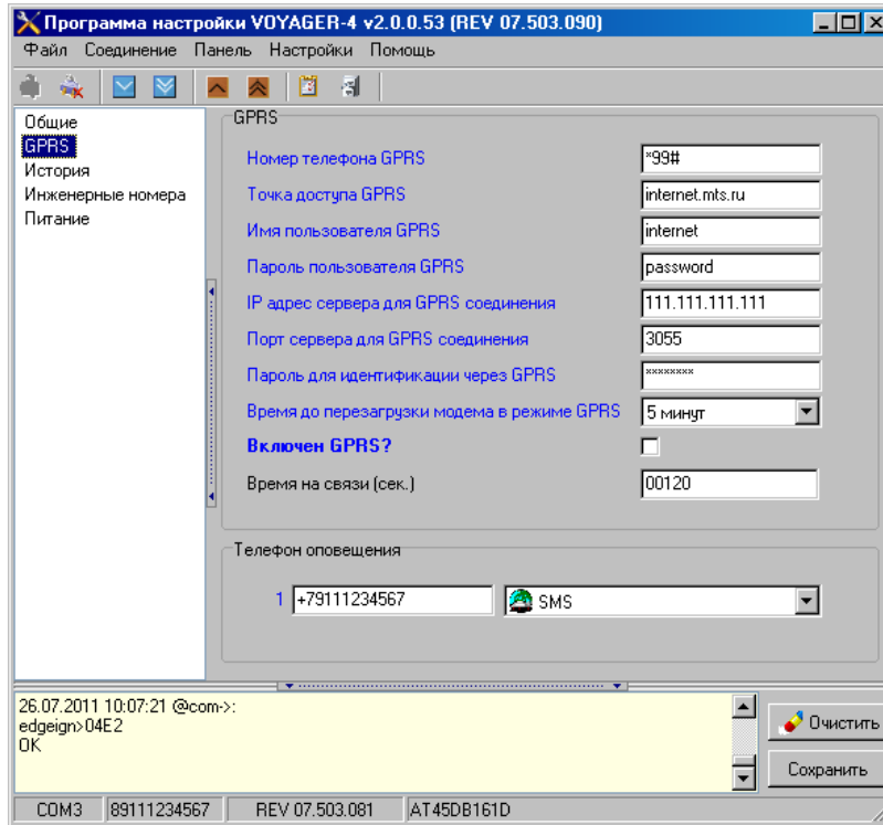
Рис.4.3.2.1. Страница настроек GPRS-соединения
