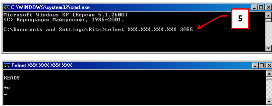
Рис.6.2. Проверка порта TCP 3055
