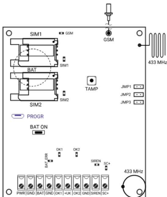
Рисунок 1. Панель охранно-пожарная “Контакт GSM-14A.v3”
